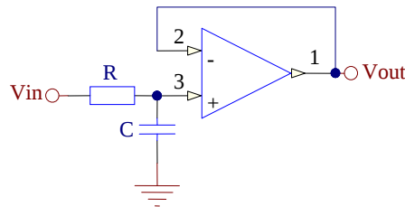
图 1 有源滤波
