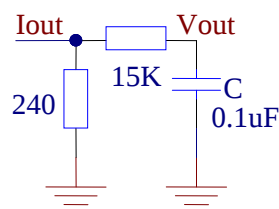
图 1 滤波电路
